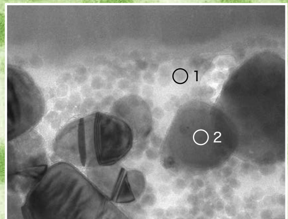
ナノコンポジットWの塗膜断面図
